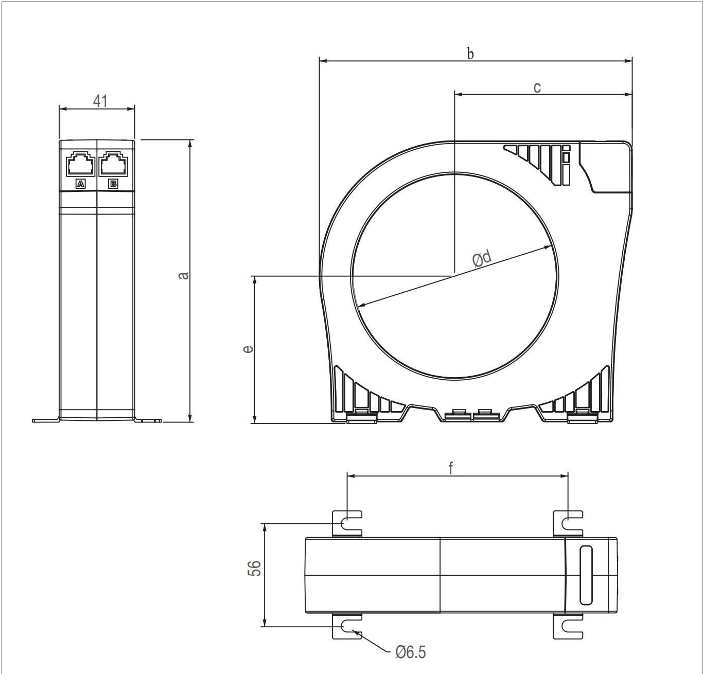
Afbeelding 48 : Afmetingen van de HR72x
