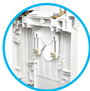
Praktische kabeldoorvoer in de sokkel
