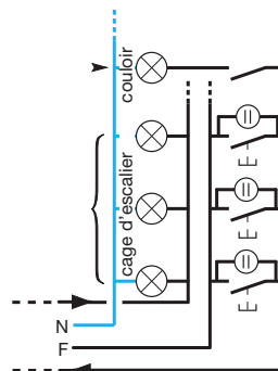
Schéma 4 fils
