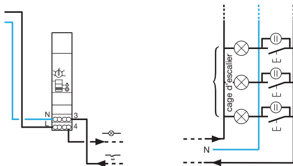
Schéma 3 fils
