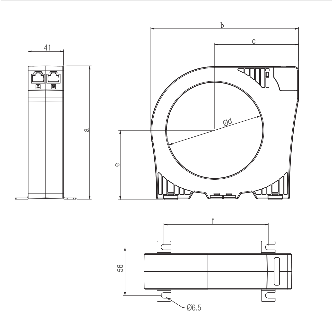
Image 48 : Dimensions du HR72x
