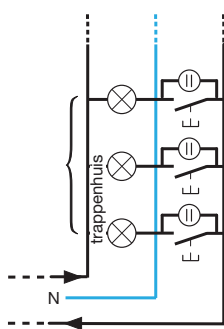
Schema - 3-draads
