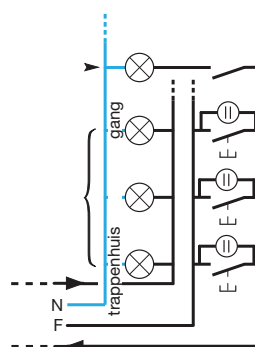
Schema - 4-draads
