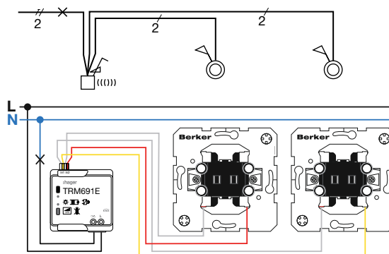
Εικόνα 3: Συνδεσμολογία για ρύθμιση φωτισμού ενός φωτιστικού, σύνδεση εισόδων με μπουτόν
