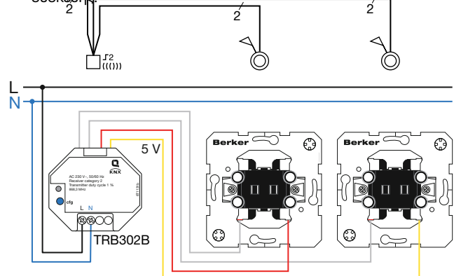
Εικόνα 4: Λειτουργία με μπουτόν (επαφές NO)
