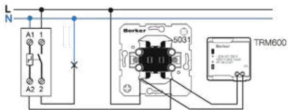
Εικόνα 1: Συνδεσμολογία με μπουτόν και αυτ.κλιμακοστάσιο
