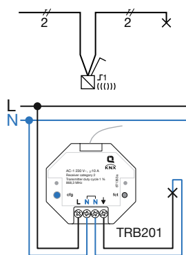
Εικόνα 2: Έλεγχος 1 φωτιστικού
