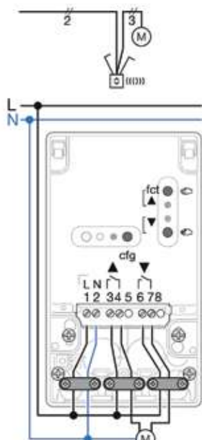
Εικόνα 1: Συνδεσμολογία ελέγχου μοτέρ ρολών
