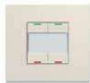
dune
