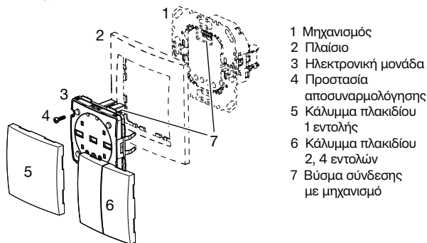
Εικόνα 1: Σύνθεση ασύρματων διακοπών
