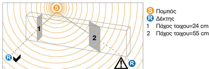
Εικόνα 3: Πάχος τοίχου για αποτελεσματική διάδοση σημάτων
