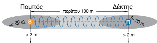
Εικόνα 1: Αποστάσεις πηγών παρεμβολών σε ελεύθερο πεδίο
