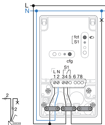
Εικόνα 2: Συνδεσμολογία για έλεγχο 1 φωτιστικού
