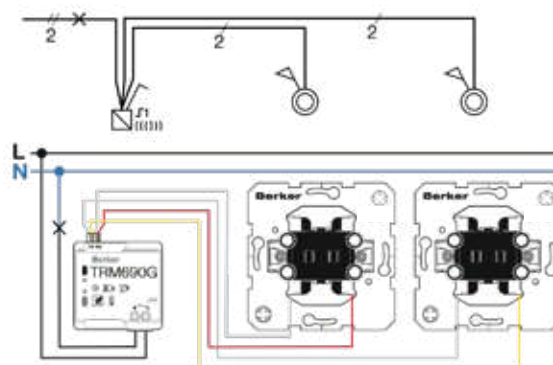
Εικόνα 3: Έλεγχος 1 φωτιστικού, σύνδεση εισόδων με μπουτόν
