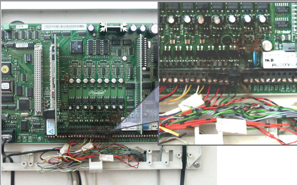
Ejemplos de material destruido por las sobretensiones transitorias.
